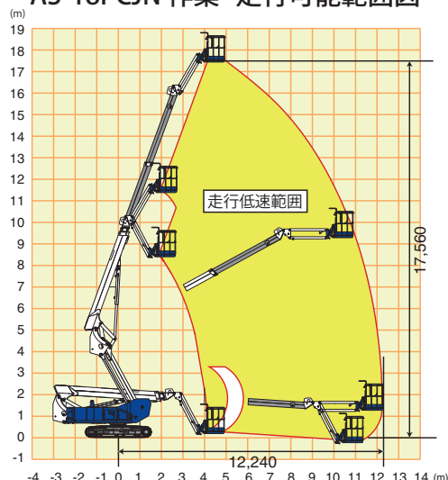
AS-18PCJN 作業・走行可能範囲図
