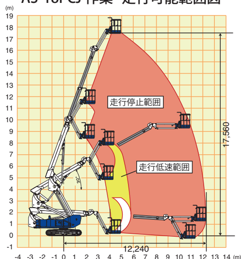
AS-18PCJ 作業・走行可能範囲図
