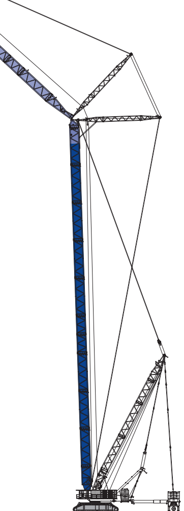
SL付きラフティングフライジブ SWSL HA 54m - 120m HI 36m - 120m
