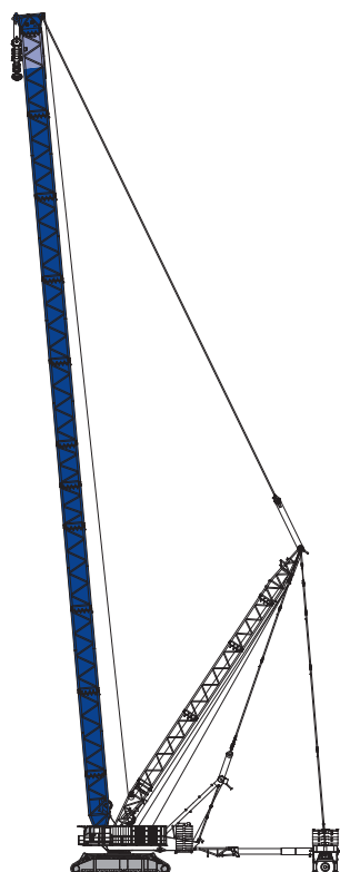
SL付きメインブーム HSSL/SSL HA 54m - 84m/120m
