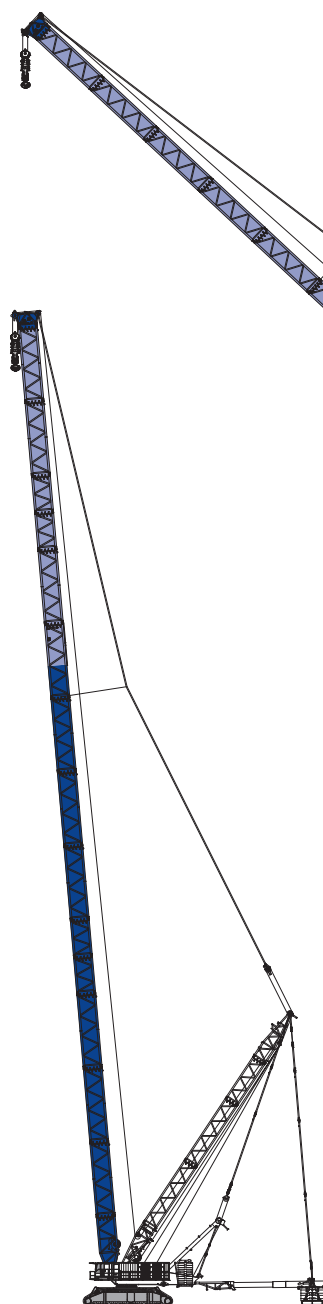
SL付きメインブーム SSL/LSL HA 114m - 156m
