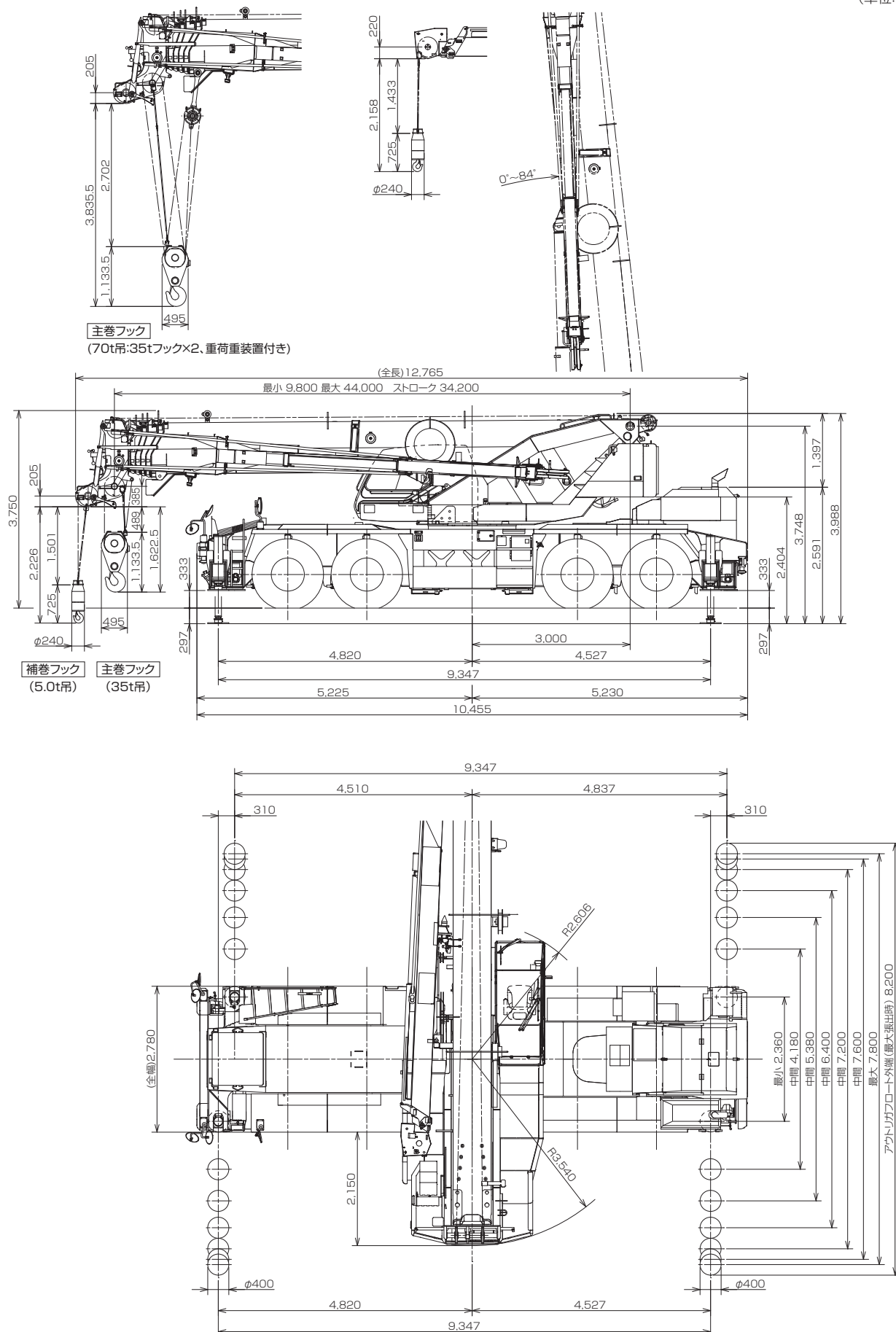
ブーム(重荷重装置取付時)
