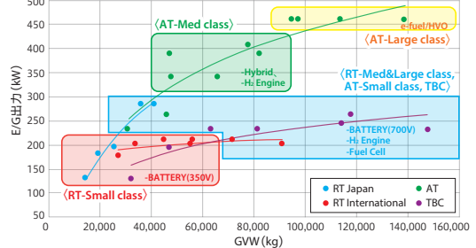
2050年カーボンネットゼロ実現に向けた中長期のクレーン動力源の方向性 GVW-E/G Output
